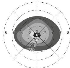
Portée de détection montage au plafond (Unité: m) Hauteur de montage proposée: 3m
