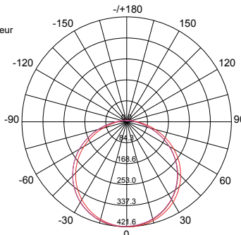
Plafondmontage (Montage plafond) Voorgestelde montagehoogte (Hauteur de montage proposée): 2,5 - 6 m
