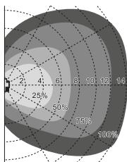
Ansbereich Wandmontage (Einheit: m) Empfohlene Montagehöhe: 2m
